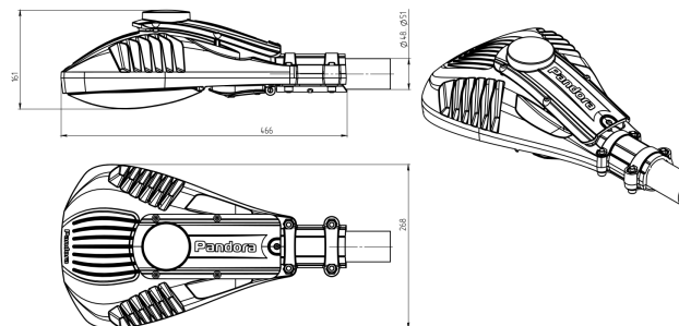
Рисунок 3. Габаритный чертеж.
